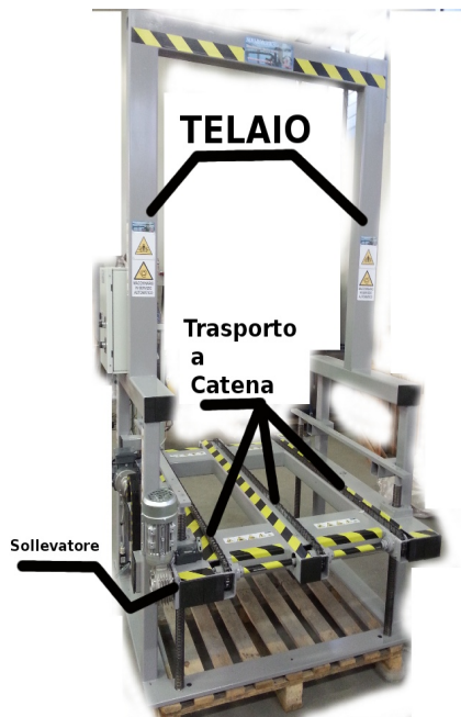
Trasporto Pallet
